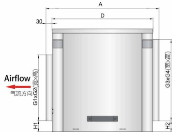
BKB200-315(0°)
