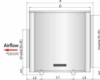
BKB355-500(0°)
